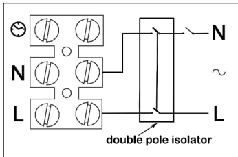
ELs - 3 Speed with Cord
