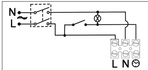
ELs - 3 Speed via remote switch
